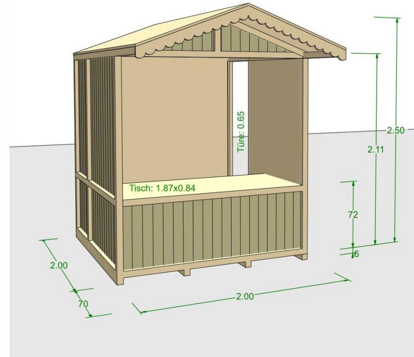
Markthäuschen 2x2m offen mit Verkaufstisch
