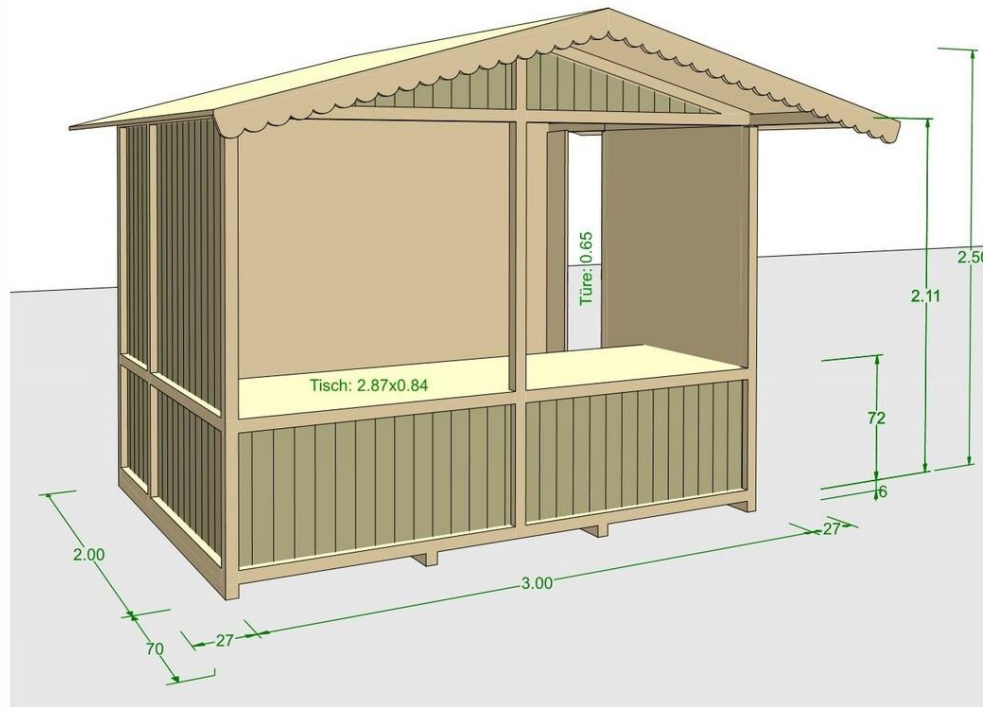
Markthäuschen 3x2m offen mit Verkaufstisch oder mit begehbare Front
